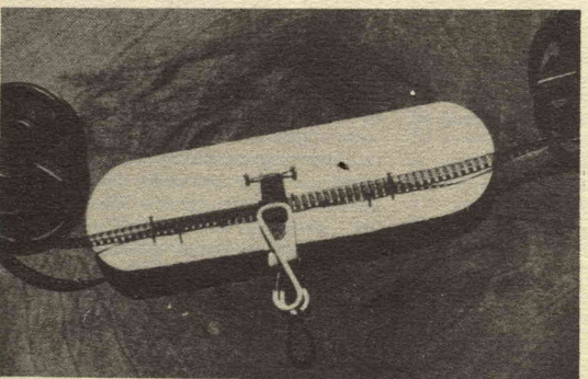
(In alto) - E' stata inserita anche la seconda estremità del film, questo è pronto per la incollatura. — (In basso) - Applicato il collante sul film, il pezzo mobile della pinzetta viene ruotato e la pinzetta viene aggiunta, per stringere il giunto.
