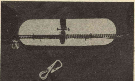
(In alto) - La pressetta pronta per l'impiego, con accanto il collante e la pinzetta che serve per esercitare la necessaria pressione. — (In basso) - La inserzione di una delle estremità del film da unire.
