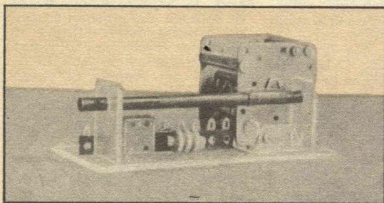
(Foto a sinistra): Ricevitore visto dal davanti: a destra le pile di Jack di uscita e l'interruttore; a sinistra si nota CV che però può essere anche del tipo « miniatura » (vedi schema pratico). — (Foto a destra): Ricevitore visto dal retro: si nota la ferrite con L avvolta, l'impedenza JAF ed altri componenti.
