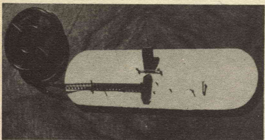
(In alto) - La pressetta pronta per l'impiego, con accanto il collante e la pinzetta che serve per esercitare la necessaria pressione. — (In basso) - La inserzione di una delle estremità del film da unire.
